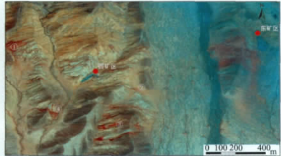
图 4 巴什布拉克东西铀矿区 Quickbird B3/B1, B2, B1 RGB 彩色合成图
