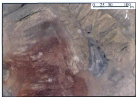
图6 巴什布拉克东矿区 Quickbird 3,2,1 多光谱波段与全色波段融合图
