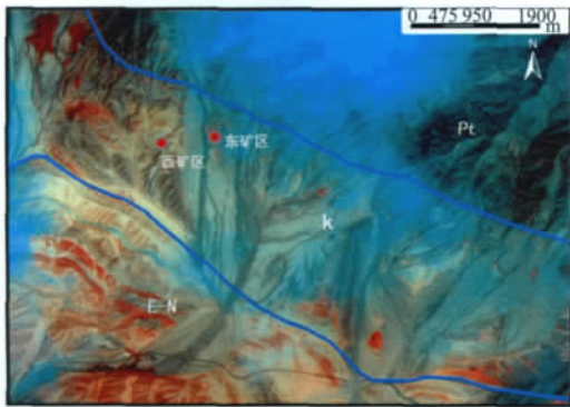
图 3 巴什布拉克铀矿区及周围 Quickbird B3/B2, B2, B1 彩色合成图
