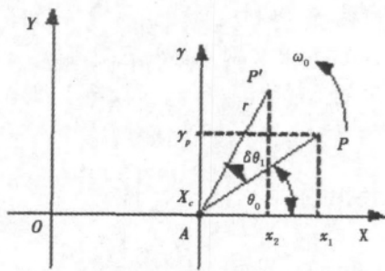
图5 目标转台模型示意图
