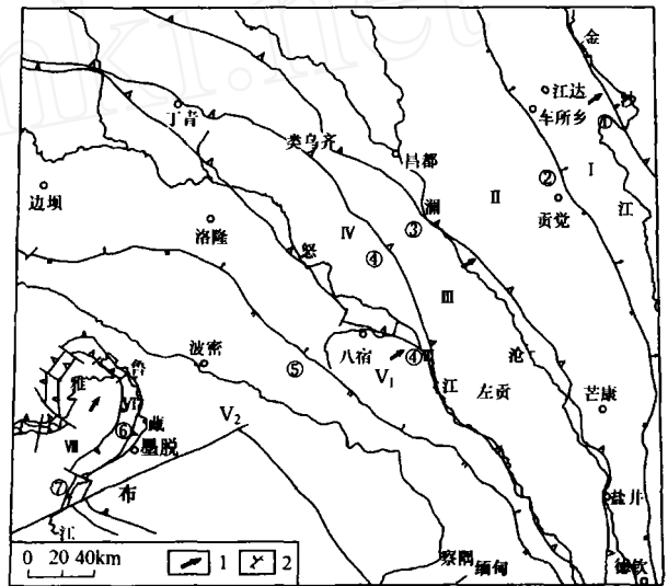
图 1 遥感解译构造纲要图
