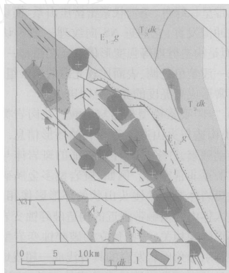
图 3 藏东弄洼优者金矿遥感五要素综合找矿远景区 1—洞卡组;2—与金矿相关成矿有利部位(其它图例同图 2)
