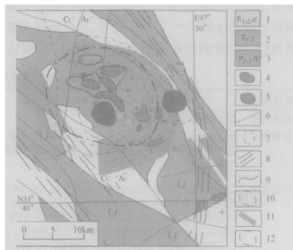
图 2 藏东包买铅锌银矿遥感五要素综合找矿远景区 1—贡觉组;2—甲丕拉组;3—宁多群;4—已知花岗岩类;5—解译花岗岩体;6—断层;7—环形构造;8—脆韧性变形带;9—不整合接触线;10—铜金化探异常区;11—与铜铅相关成矿有利部位;12—遥感找矿远景区
