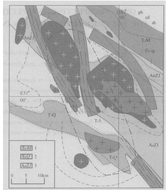
图 6 藏东打拢金矿遥感五要素综合找矿远景区 1—孟阿雄群基性火山岩; 2—确哈拉群砂岩、灰岩夹流纹岩、中基性火山岩; 3—宁多群 (其它图例同图 2)
