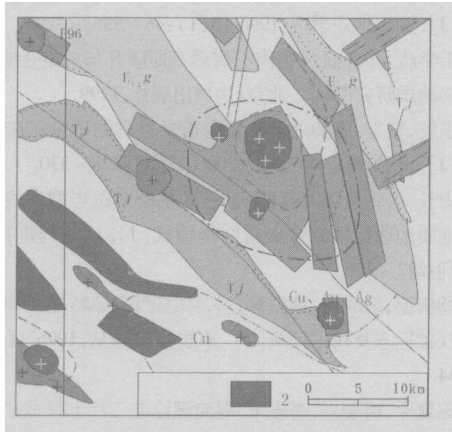
图 4 藏东瓦义勇铜金银矿遥感五要素综合找矿远景区 J 3 c—晚三叠世; 1—超基性岩; (其它图例同图 2)
