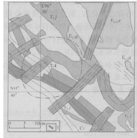
图 5 藏东卓登尔大型铅锌银矿遥感五要素综合找矿远景区 与铅锌银成矿相关有利部位 (其它图例同图 2)
