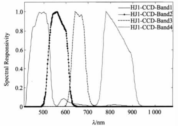
图 1 HJ-1 卫星 CCD 相机光谱响应曲线
