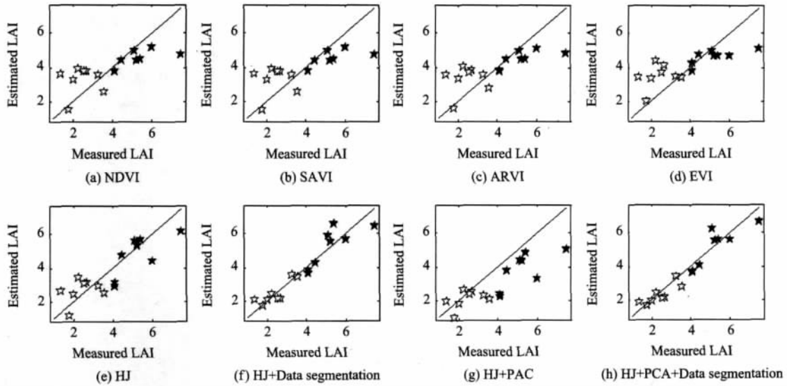
图8 以模拟 HJ-1 多光谱为数据源的预测值与实测值散点图
