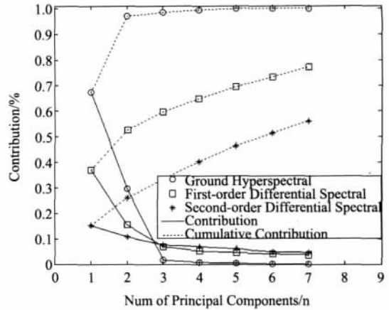
图 4 地面高光谱及其一阶、二阶微分光谱前七个主成分贡献率及累计贡献率
