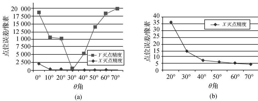
图 3 灭点误差随 \theta 角变化的曲线
