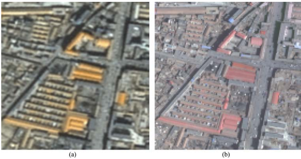
图 5 砖混结构房屋建筑震前(a)和震后(b)遥感影像 (a) 震后; (b) 震前
