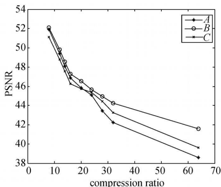
图 4 三种算法图像质量比较
