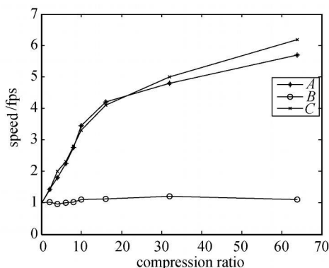
图 3 三种码率控制算法编码速度比较
