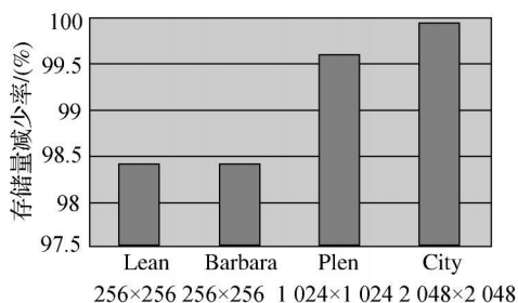
图 2 本文算法相对标准算法的存储量减少率
