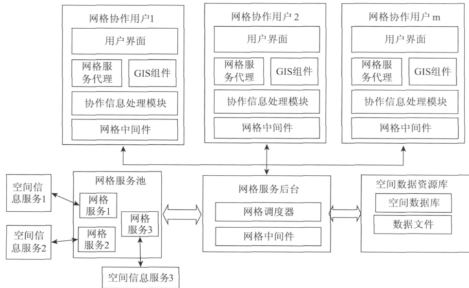
图 1 网格分布式实时协同标绘系统的框图
